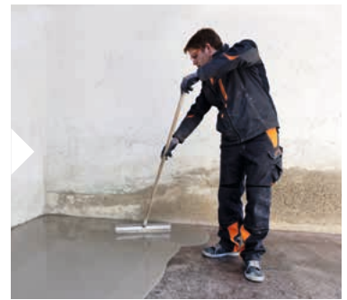
Beschichtung verteilen
